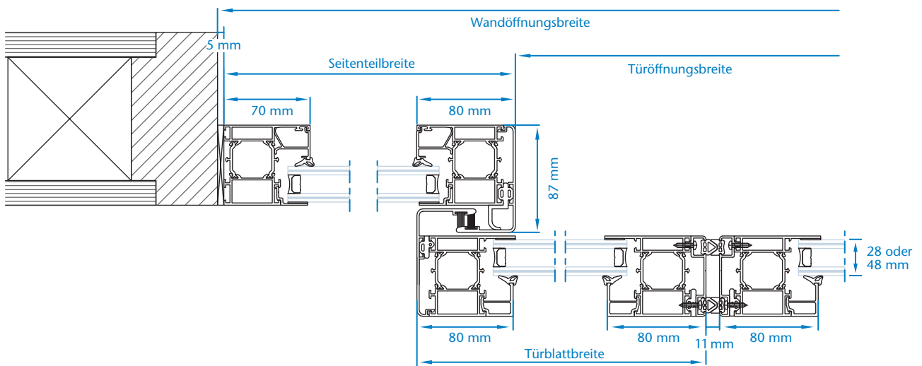
KONE SD 50 mit Isolierglas
